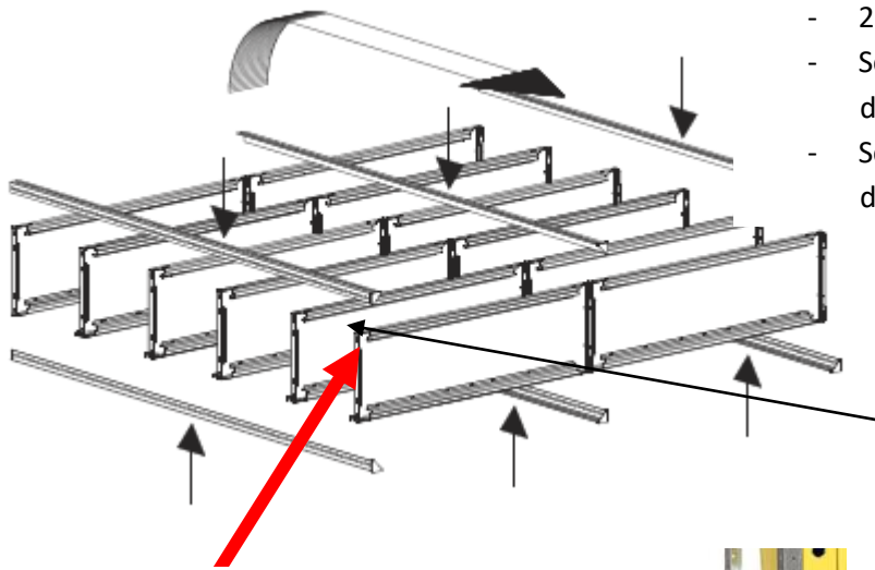
Detail der Befestigung des Regals an den Gestellbahnen
