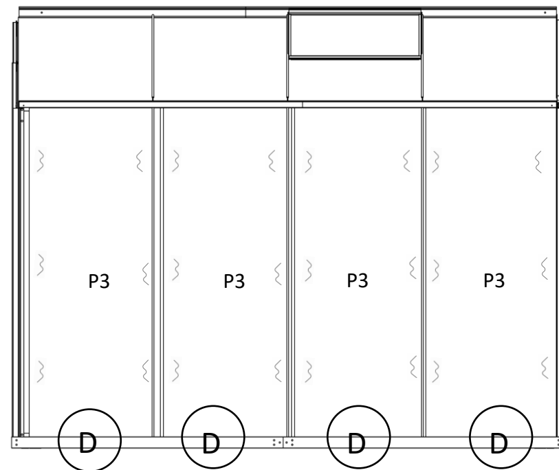
Pohled zepředu
