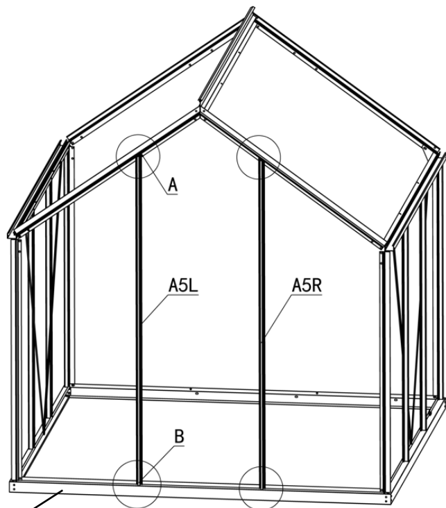
Zadní pohled
