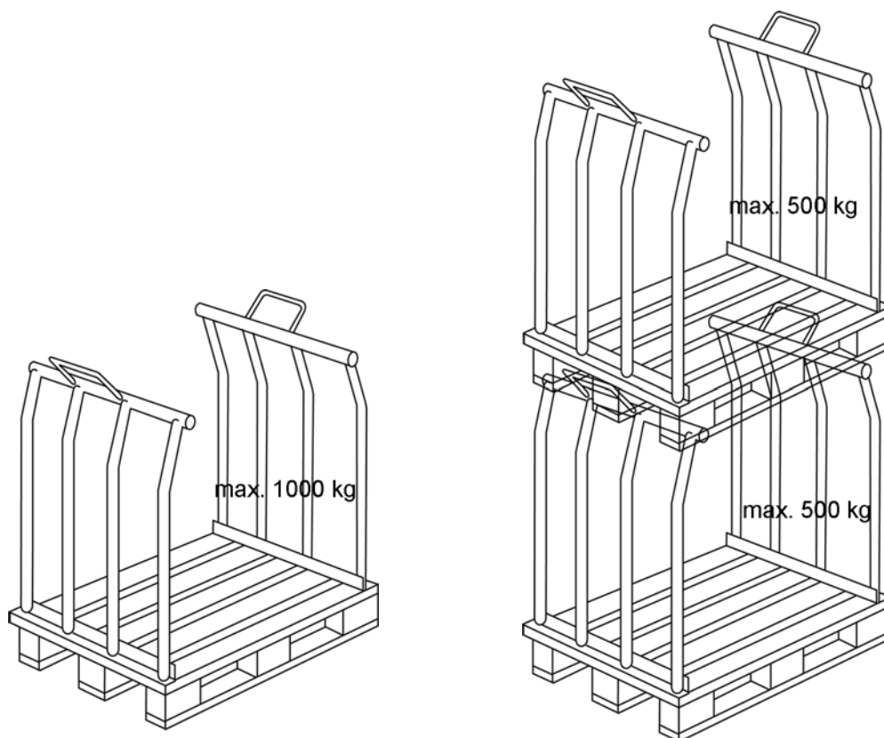
Obr. 7 nosnost při nestohování max. 1000 kg
