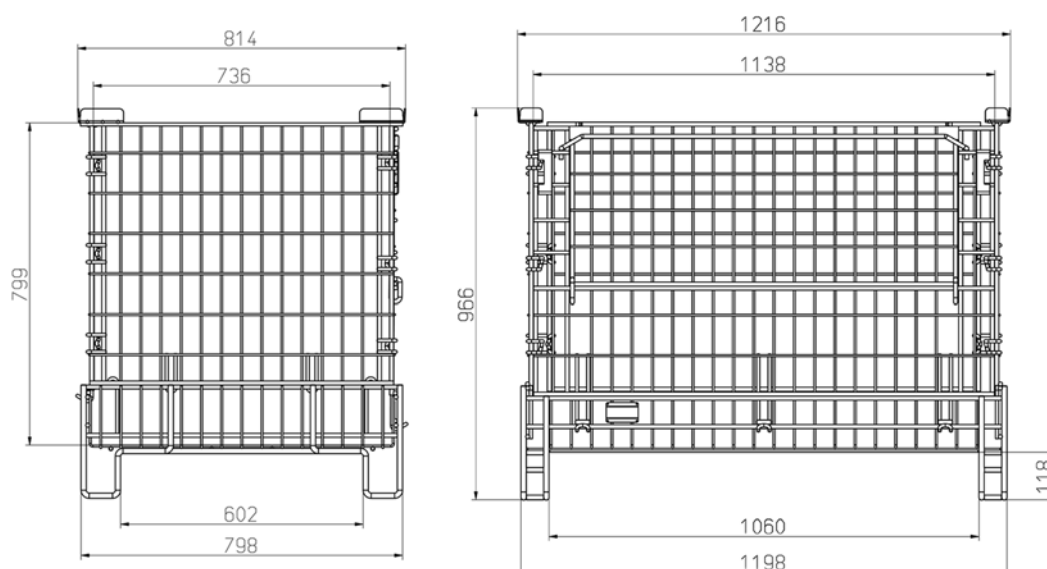
Obr. 1 PC 1000 – obj. č. 06.85390.xx-xxxx PC 1000/1 s víko - obj. č. 06.87576.xx-xxxx
