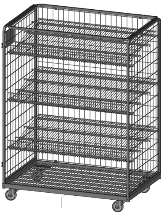
Obr. 8 Model se zadní stěnou a šikmo umístěnými policemi se zdviženými hranami
