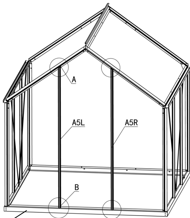
Zadní pohled
