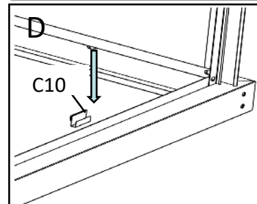
Pohled zleva
