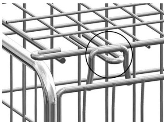
Obr. 6 Uzamčení víka se zavřenými dveřmi
