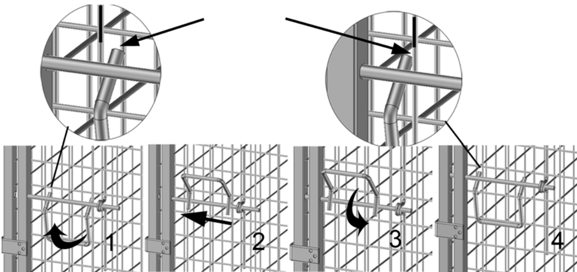
Obr. 3 Zavření dvířek
