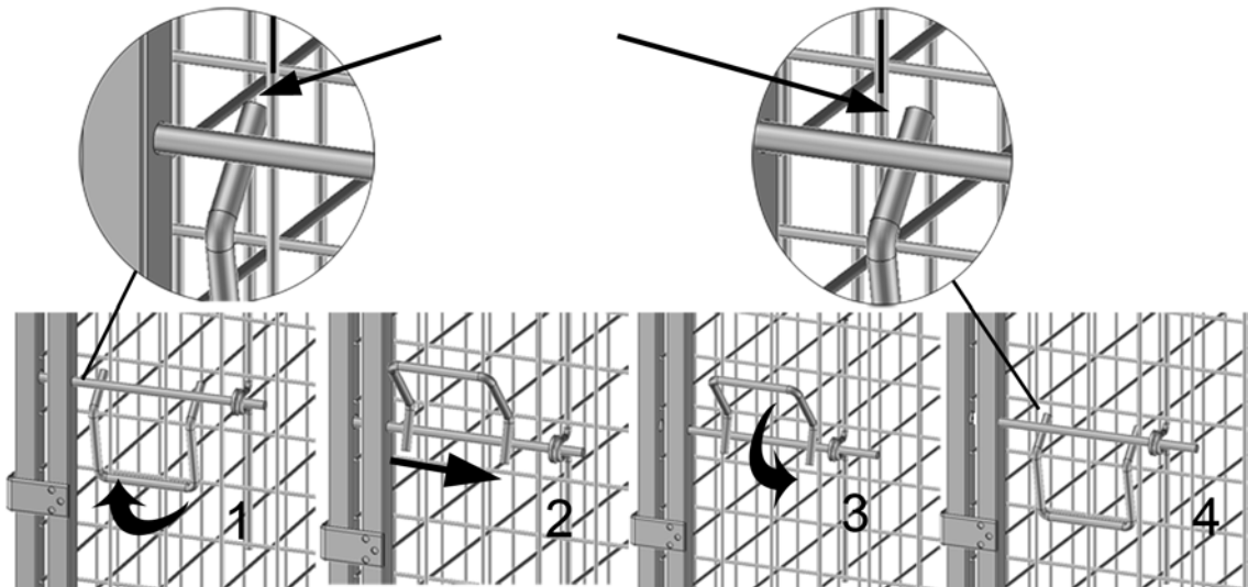
Obr. 2 Otevření dvířek
