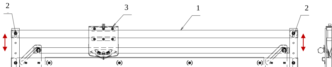
SESTAVA ŘEZÁNÍ
