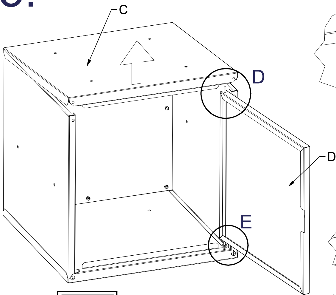
pohled zepředu
